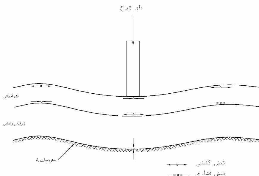
شکل ۱-۲- افت و خیز ناشی از تنشهای فشاری و کششی در روش‌سازی
