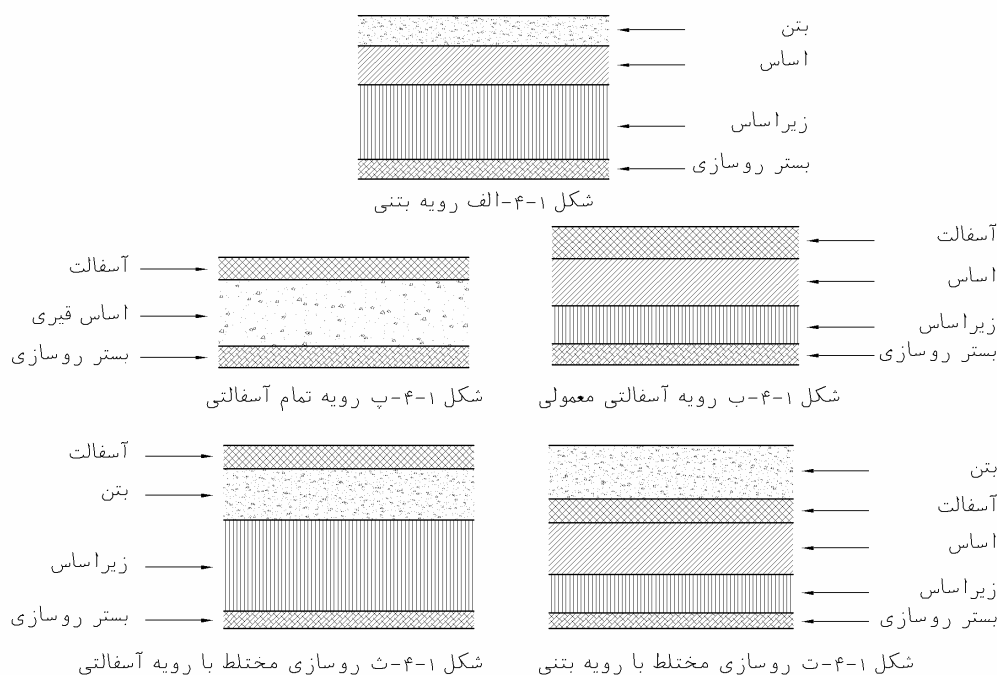
شکل ۴-۱- تیپ‌های مختلف روسازی (بتنی، آسفالتی و مختلط)
