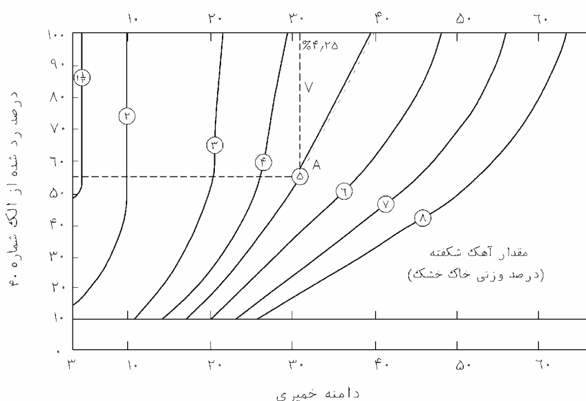
شکل ۳-۱- نمودار آشتو برای تعیین درصد آهک
