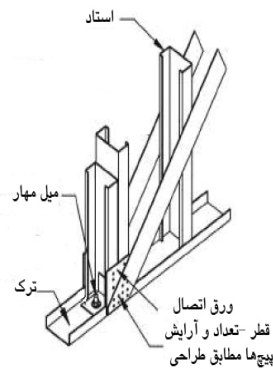
الف- اتصال مستقیم مهاربند قطری به گوشه قاب ب- اتصال مهاربند قطری به گوشه قاب به کمک ورق اتصال
