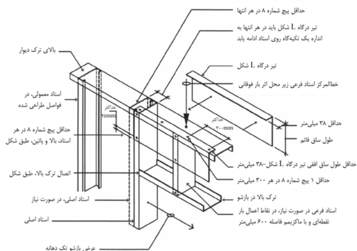
شکل ۷-۱۵ جزییات اجرای تیردرگاه به صورت مرکب متشکل از یک ترک و دو عدد نبشی سرد نورد شده
