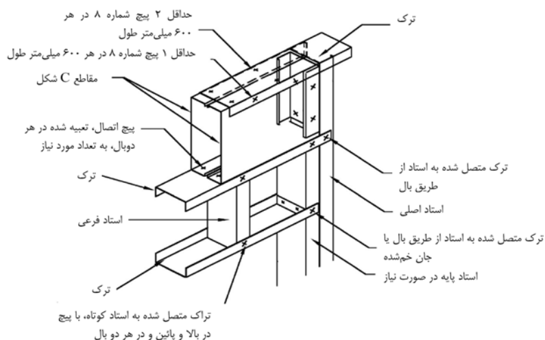
شکل ۷-۱۴: جزییات اجرای تیردرگاه به صورت مرکب متشکل از دو مقطع C شکل به صورت قوطی
