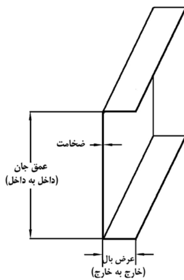
شکل ۶-۱ مقطع ترک
