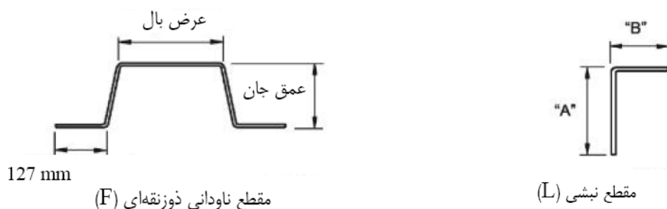
شکل ۲-۱ انواع اعضای موجود در قاب‌بندی‌های فولادی سرد نورد شده
