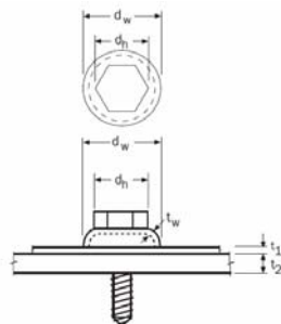
(د) واشر گنبدی زیر سرپیچ
