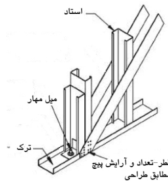
الف- اتصال مستقیم مهاربند قطری به گوشه قاب ب- اتصال مهاربند قطری به گوشه قاب به کمک ورق اتصال
