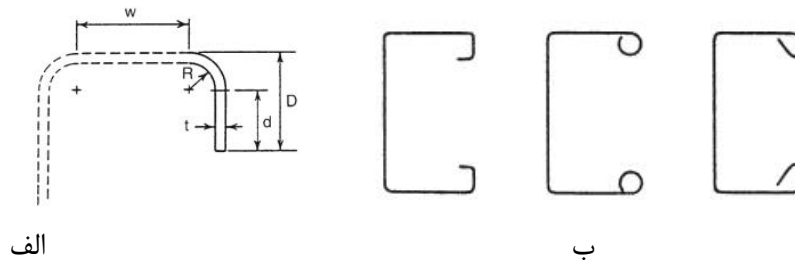
الف) سخت‌کننده لبه ساده
